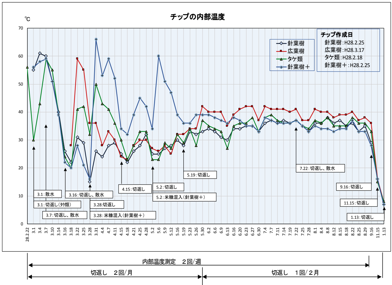
グラフA（チップの内部温度）
